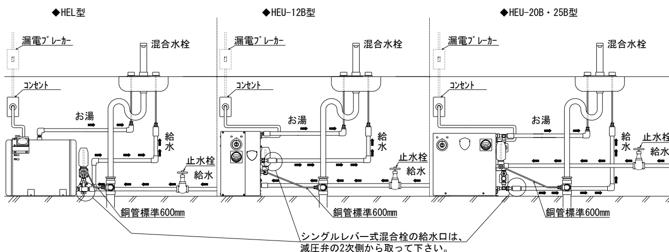
標準設置図2
