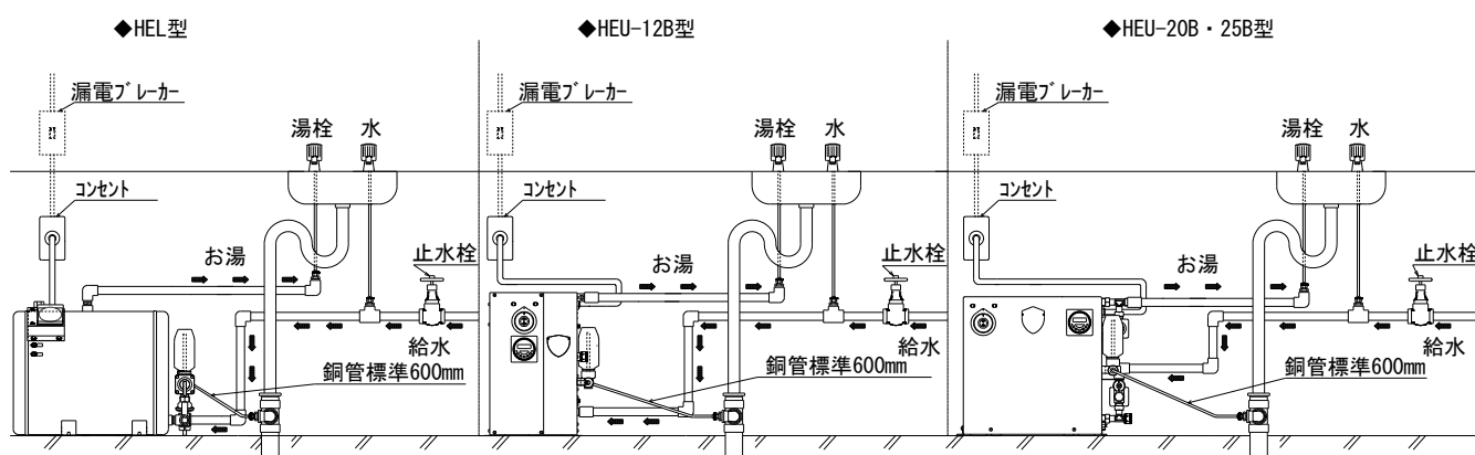
標準設置図2
