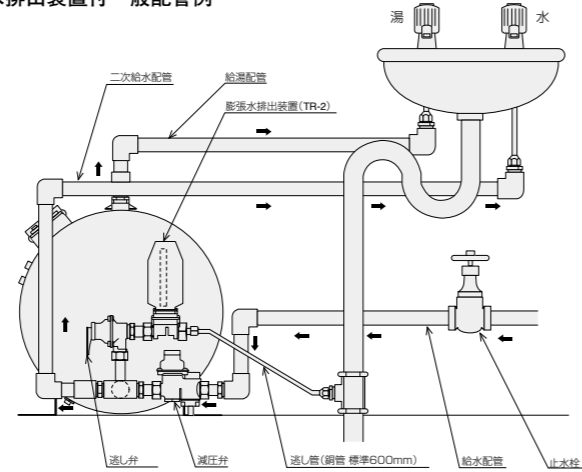
膨張水排出装置付一般配管例
